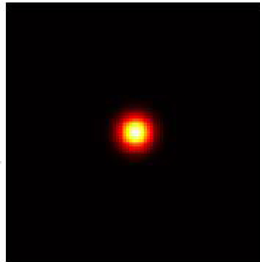
resultierender Lichtfleck
