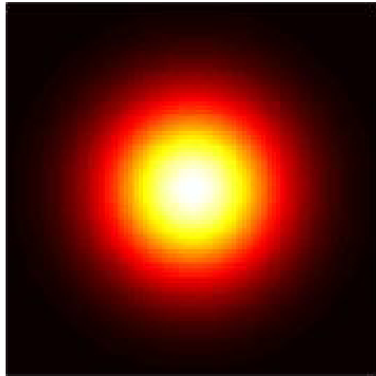
Anregungspuls
