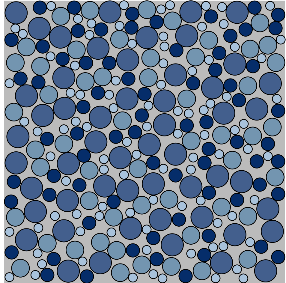
metallisches Glas
