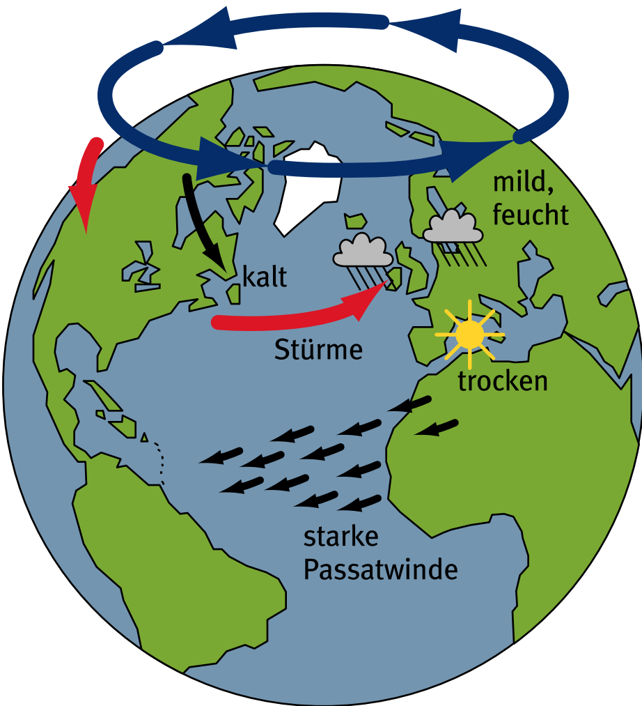
starker Stratosphärenwirbel
