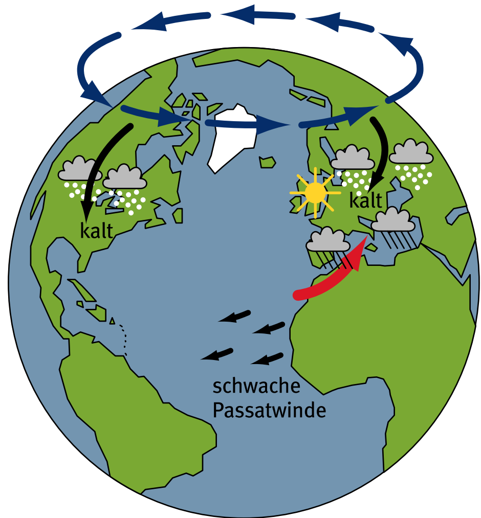
geschwächter Stratosphärenwirbel
