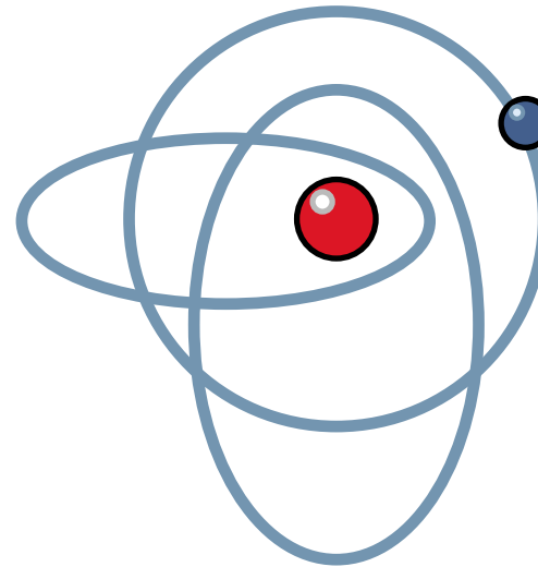
Atommodell nach Bohr und Sommerfeld
